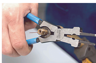
Inštalácia puzdra, montáž a demontáž.
