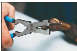
Hrot. Montáž a demontáž.
