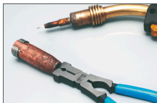
Usuwanie nagaru i odprysków z końcówki dyszy
