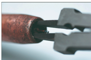
Rimozione delle scorie dall'estremità del bocchello
