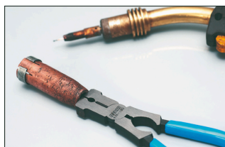
A fúvóka peremén megtapadt szennyeződés eltávolítása
