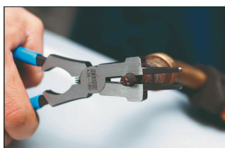
Démontage et remontage du tube contact
