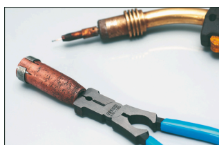
Nettoyage des éclaboussures sur la buse
