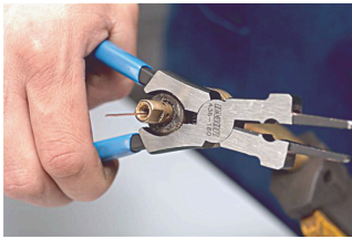
Düsenstock demontieren und montieren
