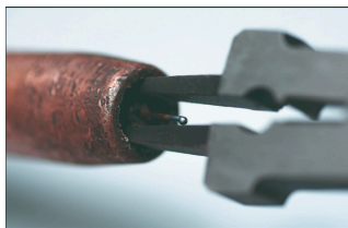
entfernen der Schweißspritzer inner bzw. Ausserhalb der Gasdüse
