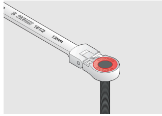
Anahtarın halka kısmındaki durdurma halkası, anahtarın somundan beklenmedik bir şekilde kaymasını önler ve tekrar somuna konumlandırılmasını sağlar.
