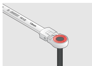
"zaustavni" prsten na okastom dijelu ključa spriječava proklizavanje ključa s matice i pozicionira ga nazad na maticu
