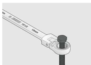
bez zaustavnog prstena
