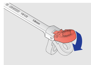
omogućava rad sa nagibom prstena glave do max. 90°
