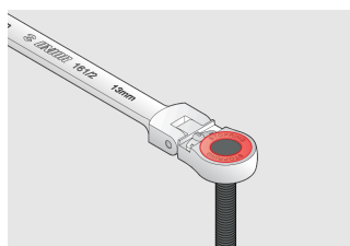
Ο δακτύλιος ασφαλείας στην πλευρά του πολύγωνου αποτρέπει το αιφνίδιο γλύστρημα από το παξιμάδι
