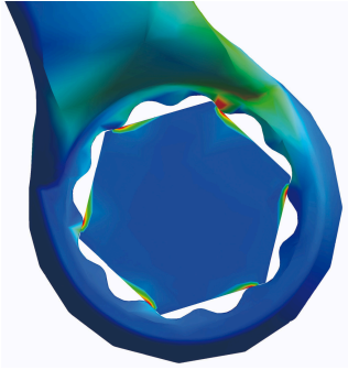
profil LIFE
